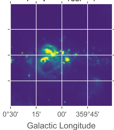
plt.style.use('ggplot')
