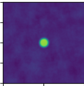
TrapezoidDisk2DKernel
