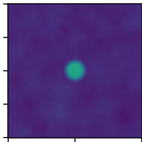
TrapezoidDisk2DKernel
